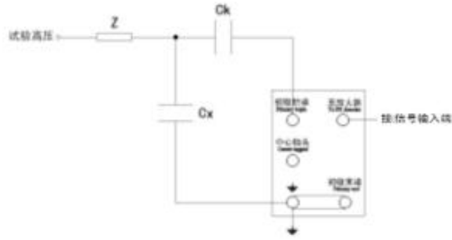
图 3a 并联接法
