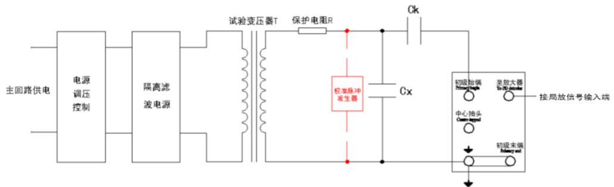
图 4 局部放电试验标准接法电路（直接法的并联法）
