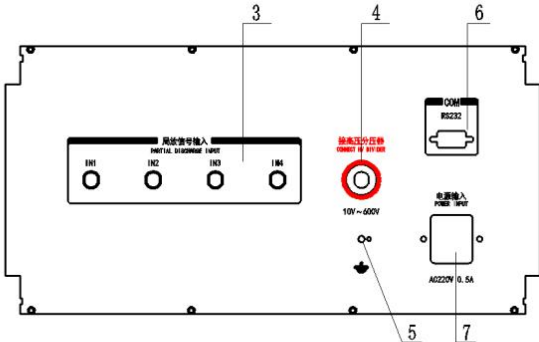
图 2b 后面板示意图
