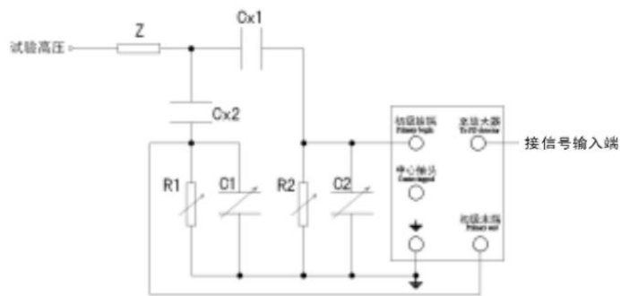
图 3d 桥式分接法
