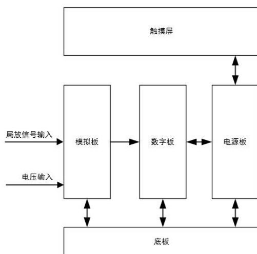
图 1 原理方框图
