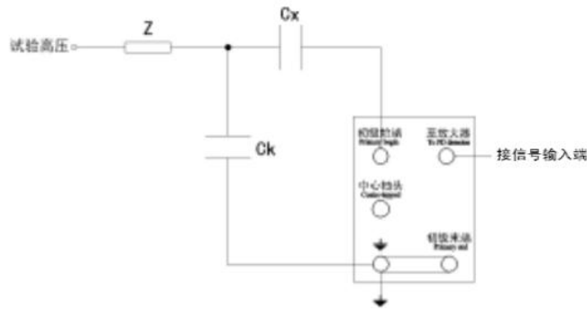
图 3b 串联接法
