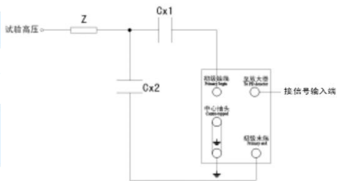
图 3c 平衡接法
